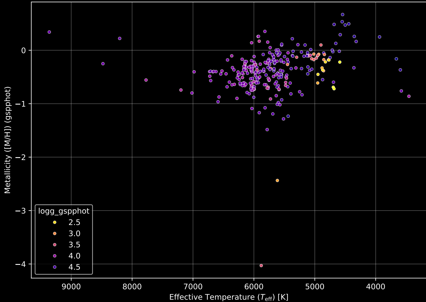
GALAH DR4 Field: [676] Stellar Population Parameters (n= 278)
