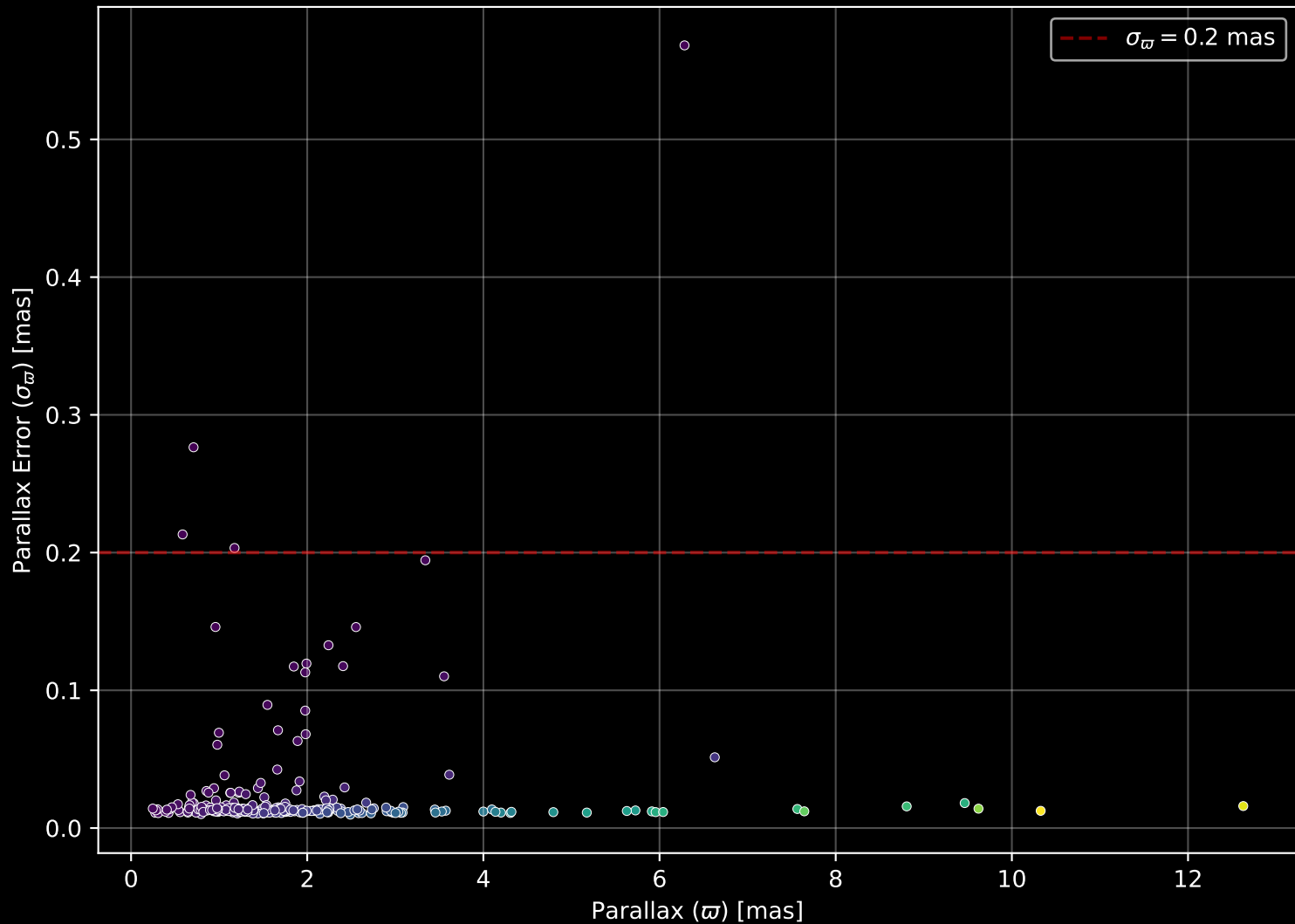
GALAH DR4 Field: [676] Parallax Quality (n= 278)
