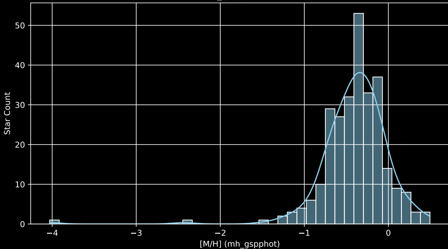
GALAH DR4 Field: [676] [M/H] (mh_gspphot) (n= 276)
