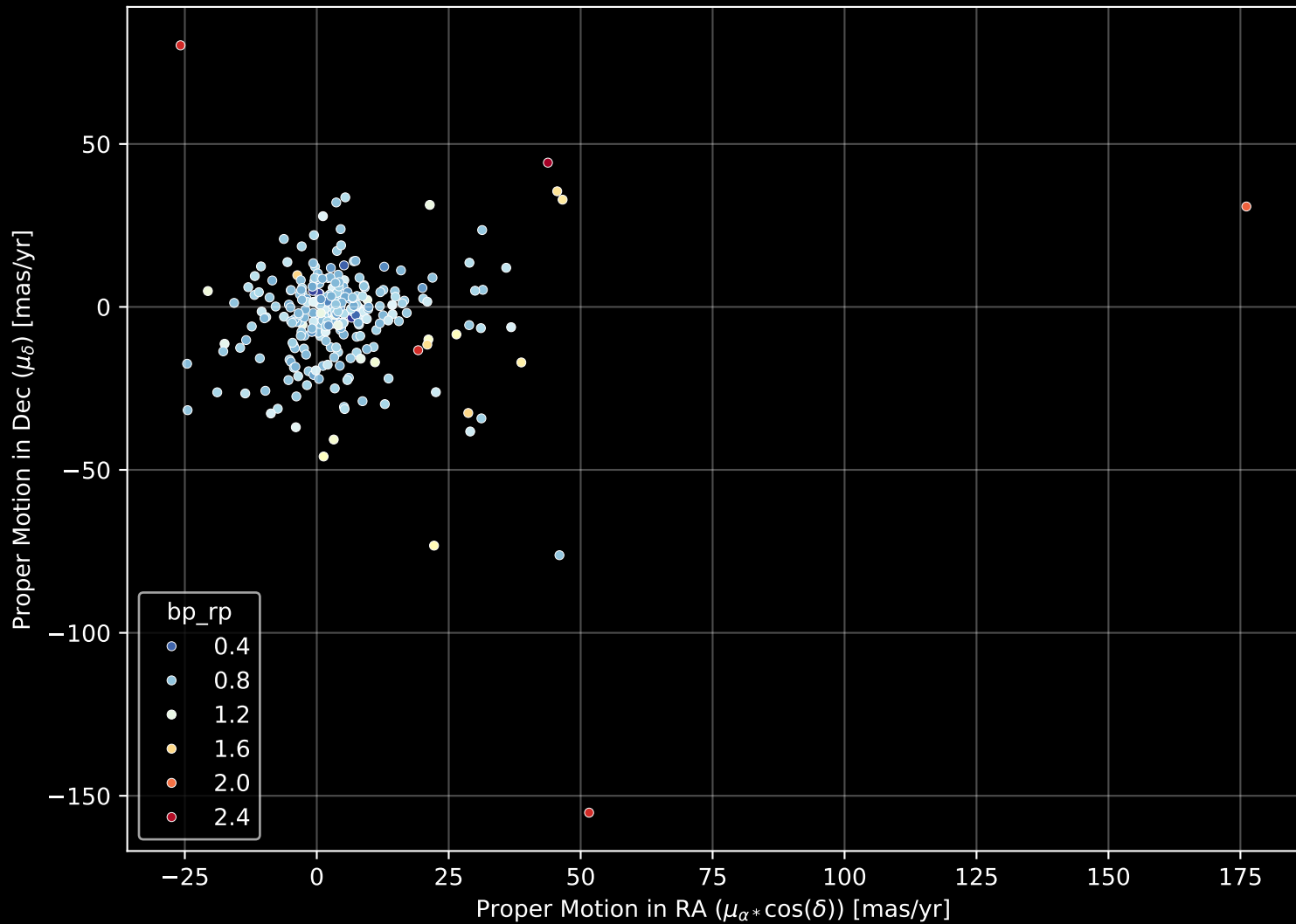
GALAH DR4 Field: [676] Proper Motion Diagram (n= 278)
